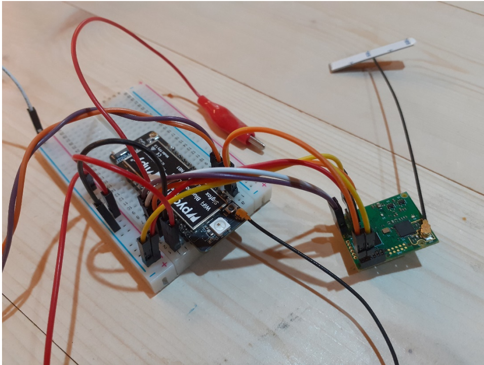
Kuva 1. Prototyypä Snapshot-paikantimesta LoPy4:llä ja Basebandin piirillä
